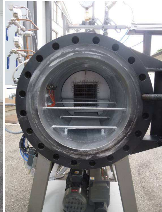
Autoclave Ø 500 x 750 a 12 BAR
