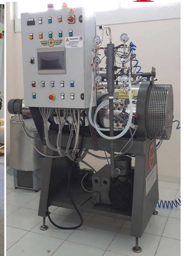
Autoclave Ø 500 x 750 a 10 BAR Autoclave Ø 550 x 800 a 13 BAR
